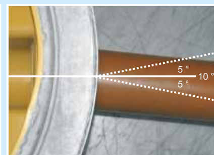
Spezielles Dichtsystem für größere Rohrabwinklung
