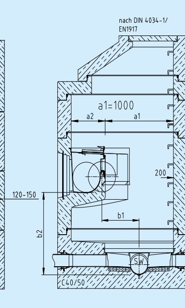
MULTRO®-HA-Schacht DN 1500
