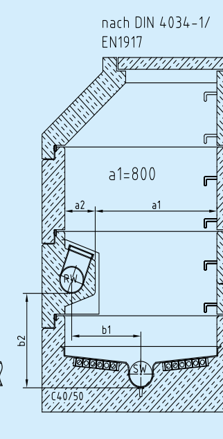
MULTRO®-HA-Schacht DN 1000
