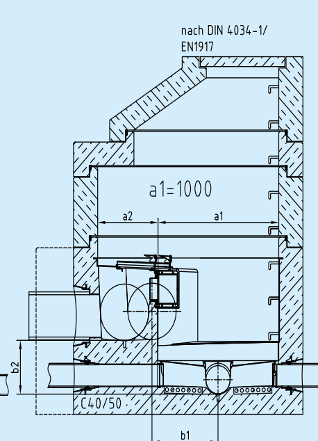
INFRA-Systemschacht DN 1500
