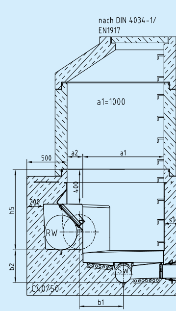
INFRA-Systemschacht DN 1200
