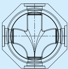
DN 150-0°/ 90°L/ 90° R
