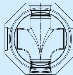
DN 200-0°/ 90°L/ 90° R
