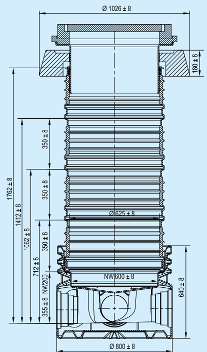
DN 200-0°/ 90°L/ 90° R
