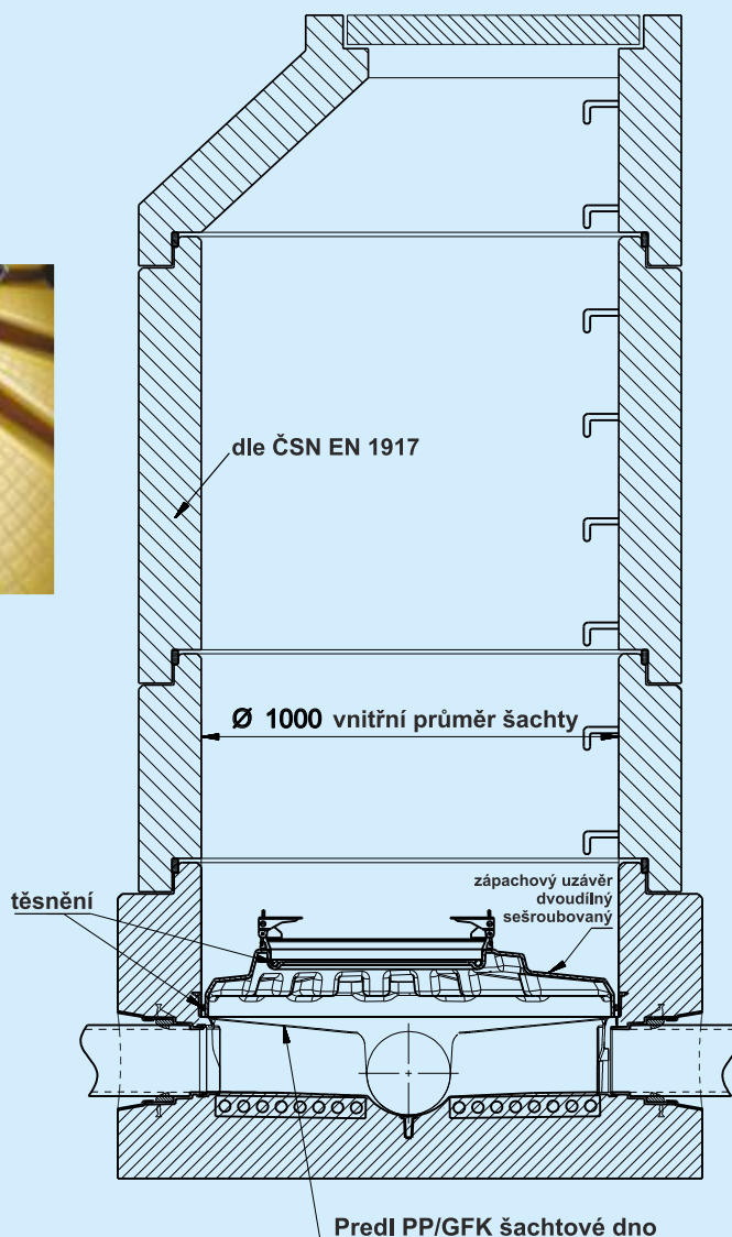
Šachta DN 1000 se zápachovým uzávěrem
