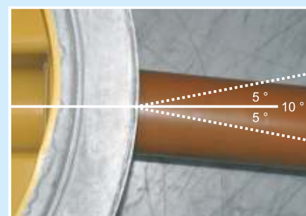
Sistema di giunzione speciale per tubi con ampie angolazioni
